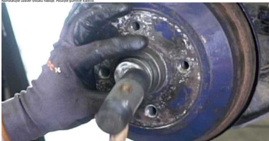
35 Natřete povrch v místě kontaktu ráfku kola s bubnovou brzdou. Použijte keramické mazivo.
