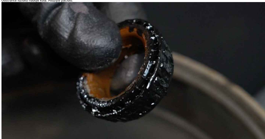
14 Vyčistěte montážní otvor ložiska náboje.
