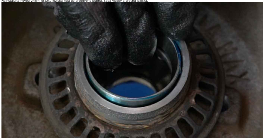
19 Nainstalujte novou vnitřní drážku ložiska kola do brzdového bubnu. Sada vložky a ořechu ložiska.
