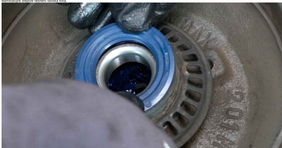
23 Natřete čep nápravy. Použijte víceúčelový čisticí sprej. Použijte mazivo na ložiska.
